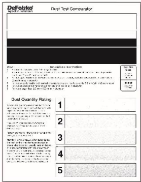
便捷灰尘测试比较卡，包括用于确定灰尘大小和灰尘量等级的图表参考
